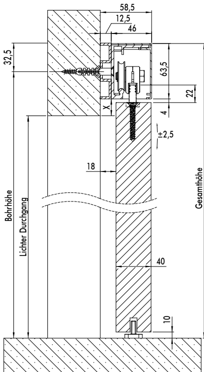
Holztürhöhe = Gesamthöhe - 63,5 - 4 - 10 mm X = Überstand
